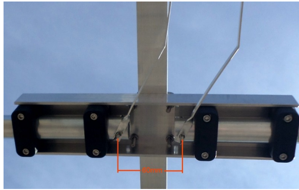
Profil U80x40mm
