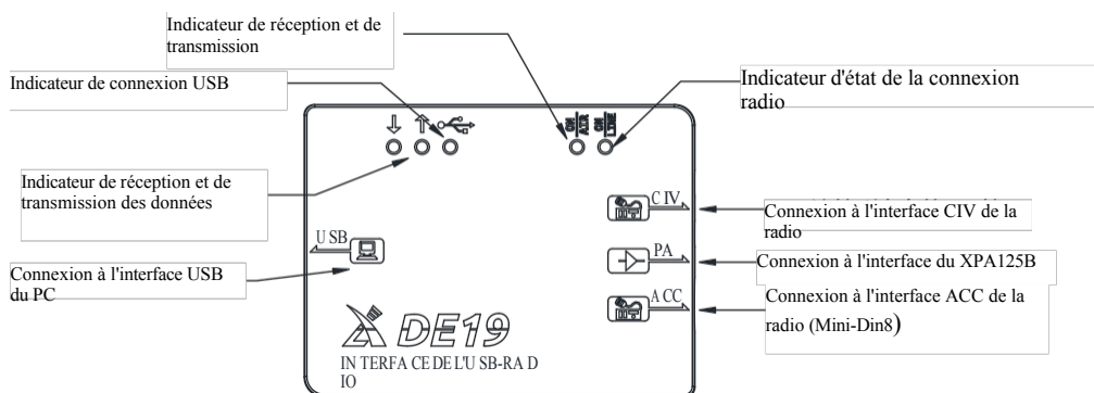
Fig. 1 Description de l'interface DE-19
