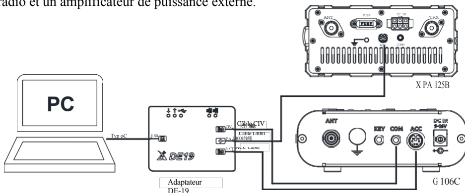
Fig. 2 Schéma de connexion entre DE-19 et G106C/XPA125B
